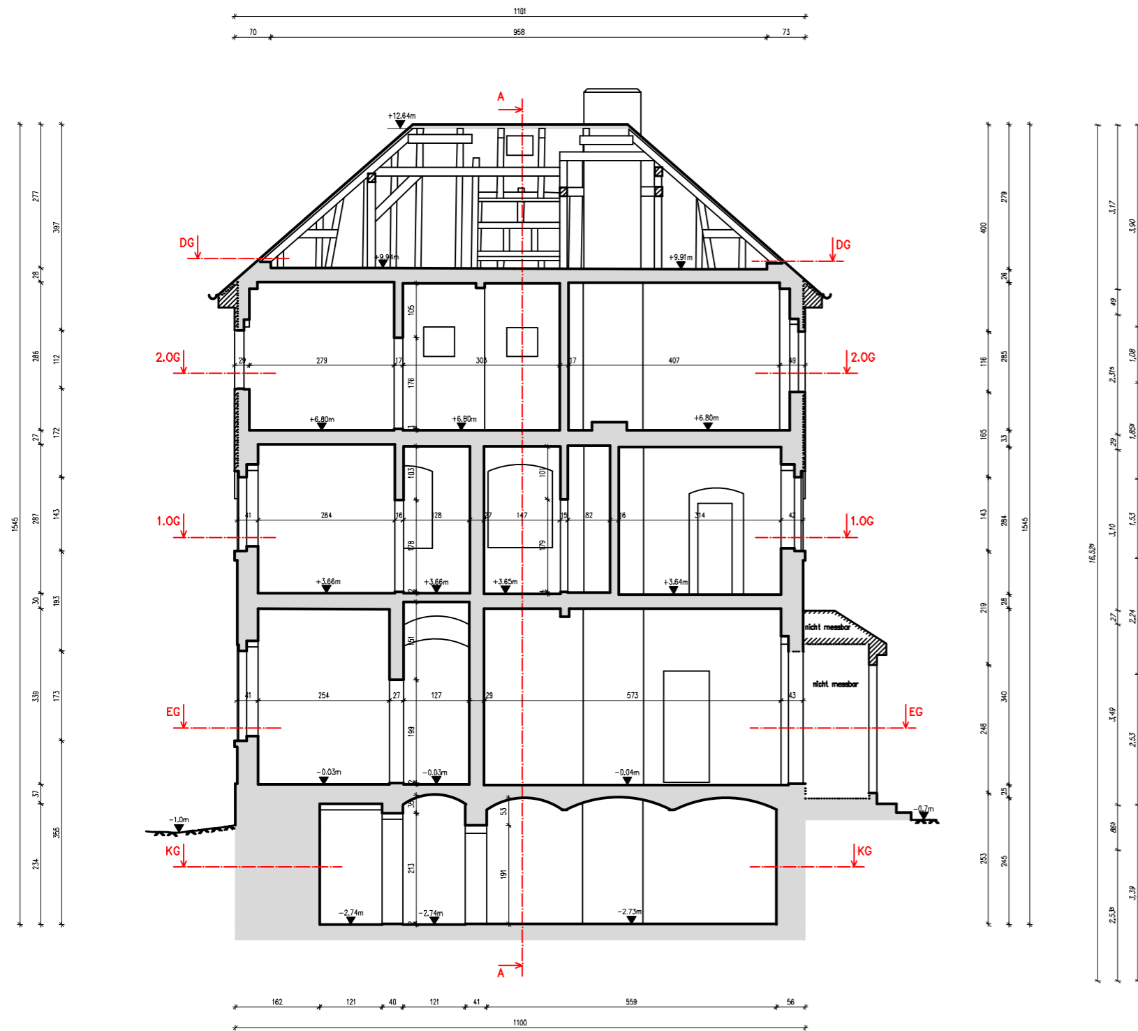
Beispiel eines geometrischen Aufmaßes
