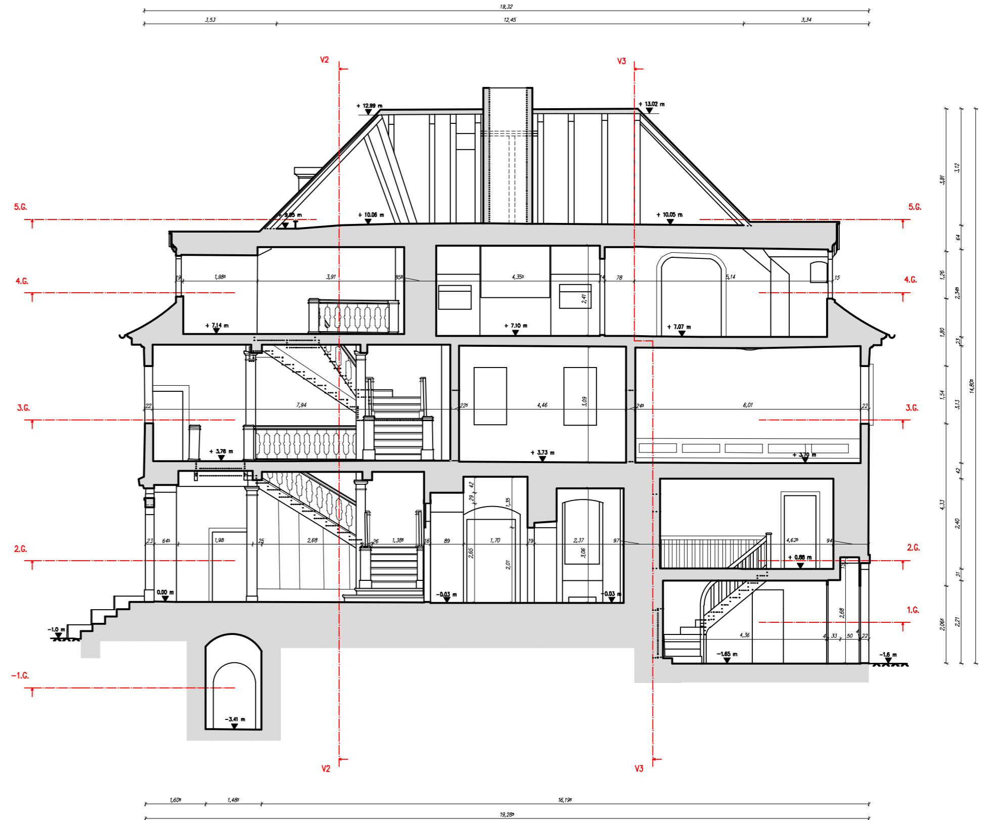
Beispiel eines verformungsgerechten Aufmaßes
